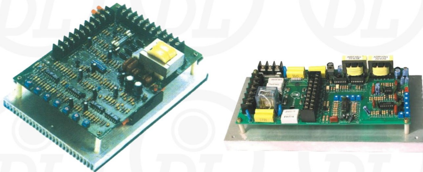
DC SCR CONTROL 無外殼式標準規格
